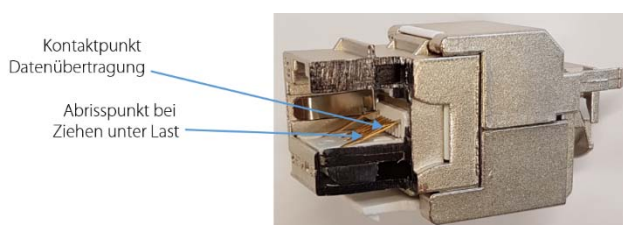
Schnitt eines RJ45-Moduls (Buchse) im Bereich der Kontaktfedern
