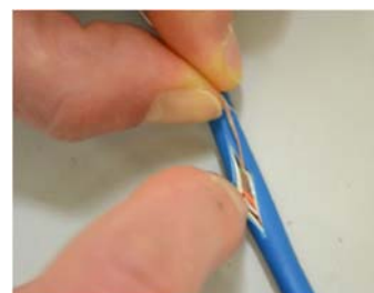
Platzierung eines Thermoelements im Kabel und des Kabels im Bündel
